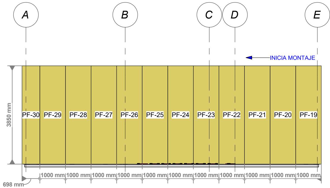
1 Fachada 2 P-04 1 : 75
