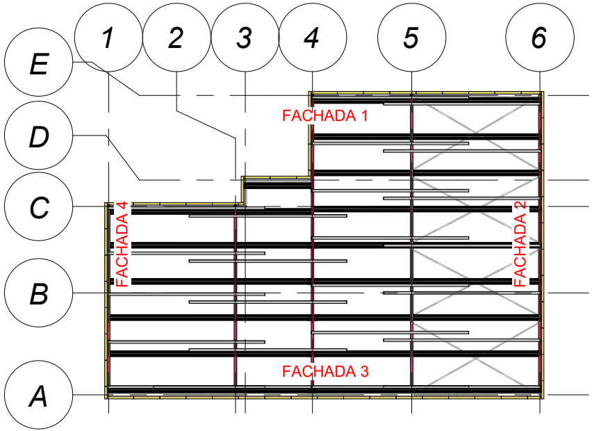
3 Referencia 1 P-03 1 : 200
