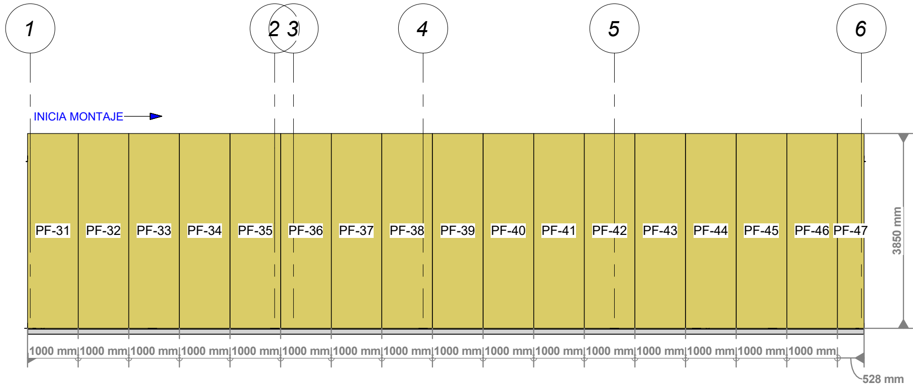
1 Fachada 3 P-05 1 : 75
