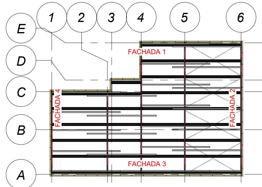
3 Referencia 3 P-05 1 : 200
