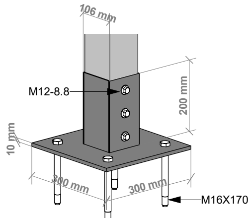
DETALLE REFUERZO 30
