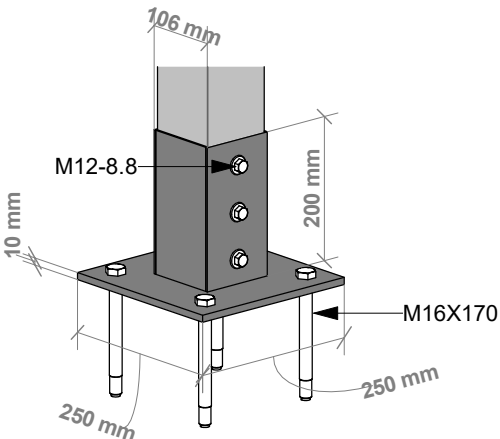
DETALLE REFUERZO 25
