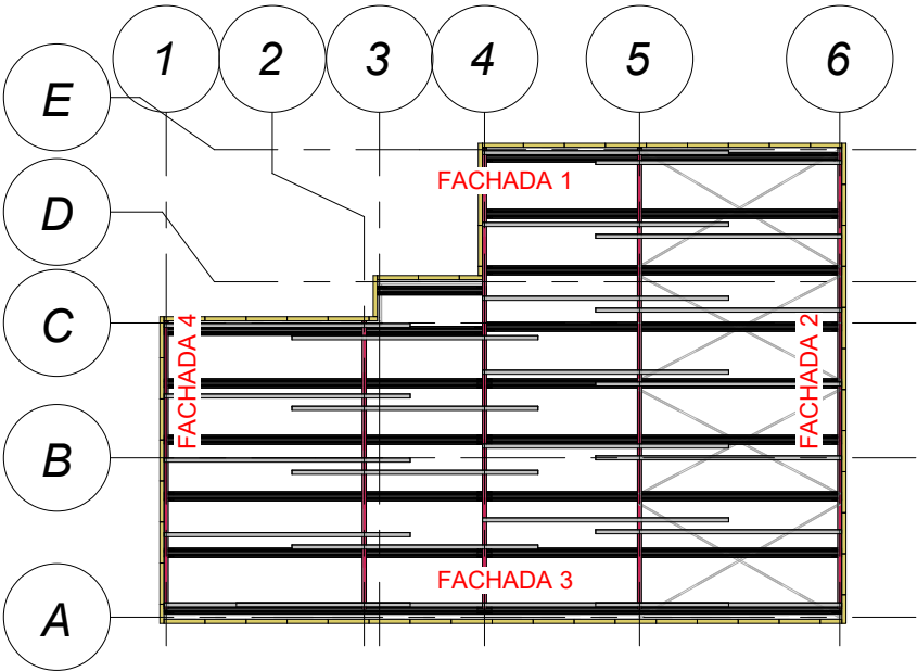
3 Referencia 2 P-04 1 : 200
