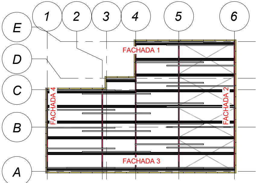
3 Referencia 4 P-06 1 : 200
