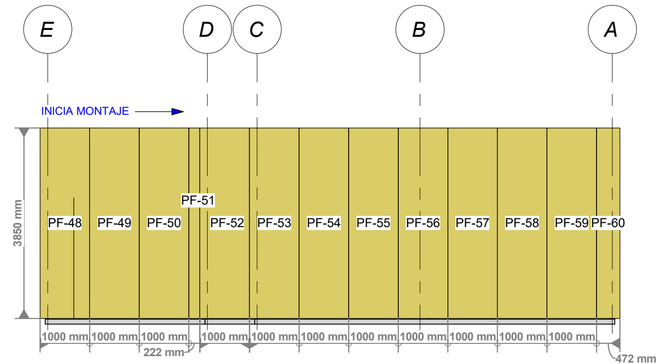
1 Fachada 4 P-06 1 : 75
