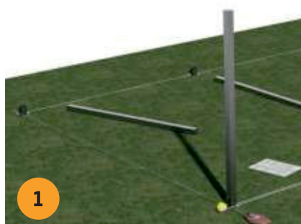
Replanteo y premontaje de los pilares en las piezas de anclaje al suelo.
