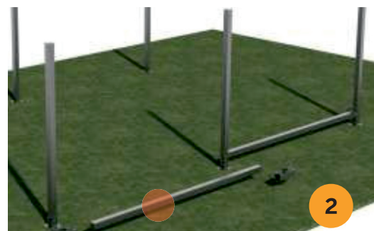
Montaje del zuncho perimetral inferior
