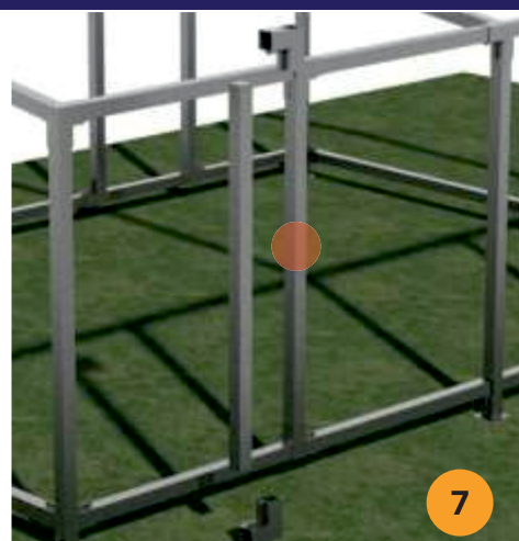
Montaje de las piezas especiales para la formación de los marcos de puertas y de las ventanas
