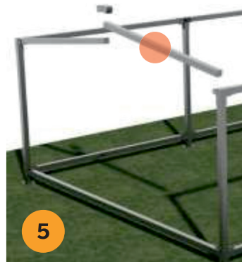
Montaje del Perímetro de cubierta, y formación de las dos aguas
